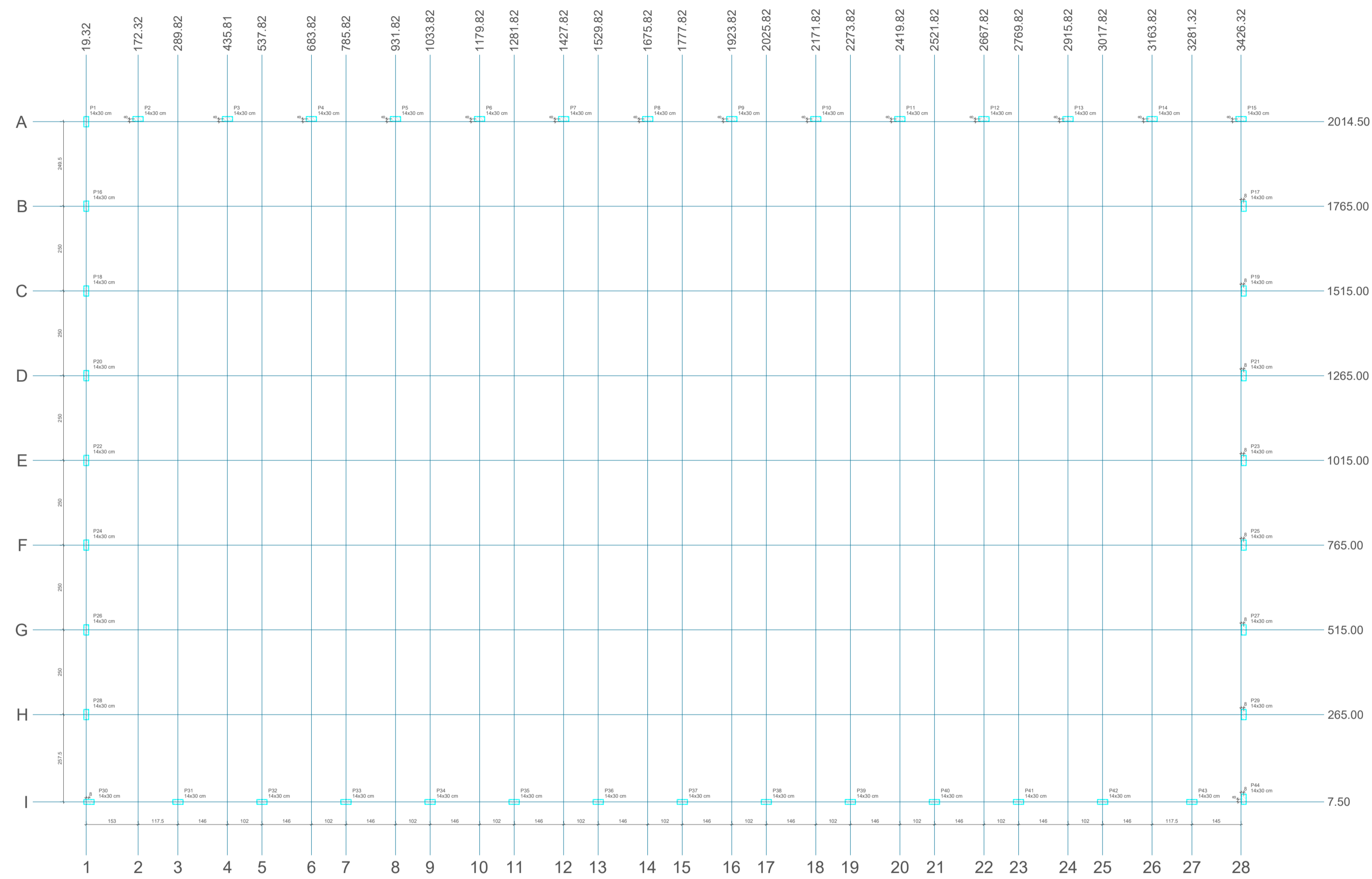
Planta de cargas escala 1:50
