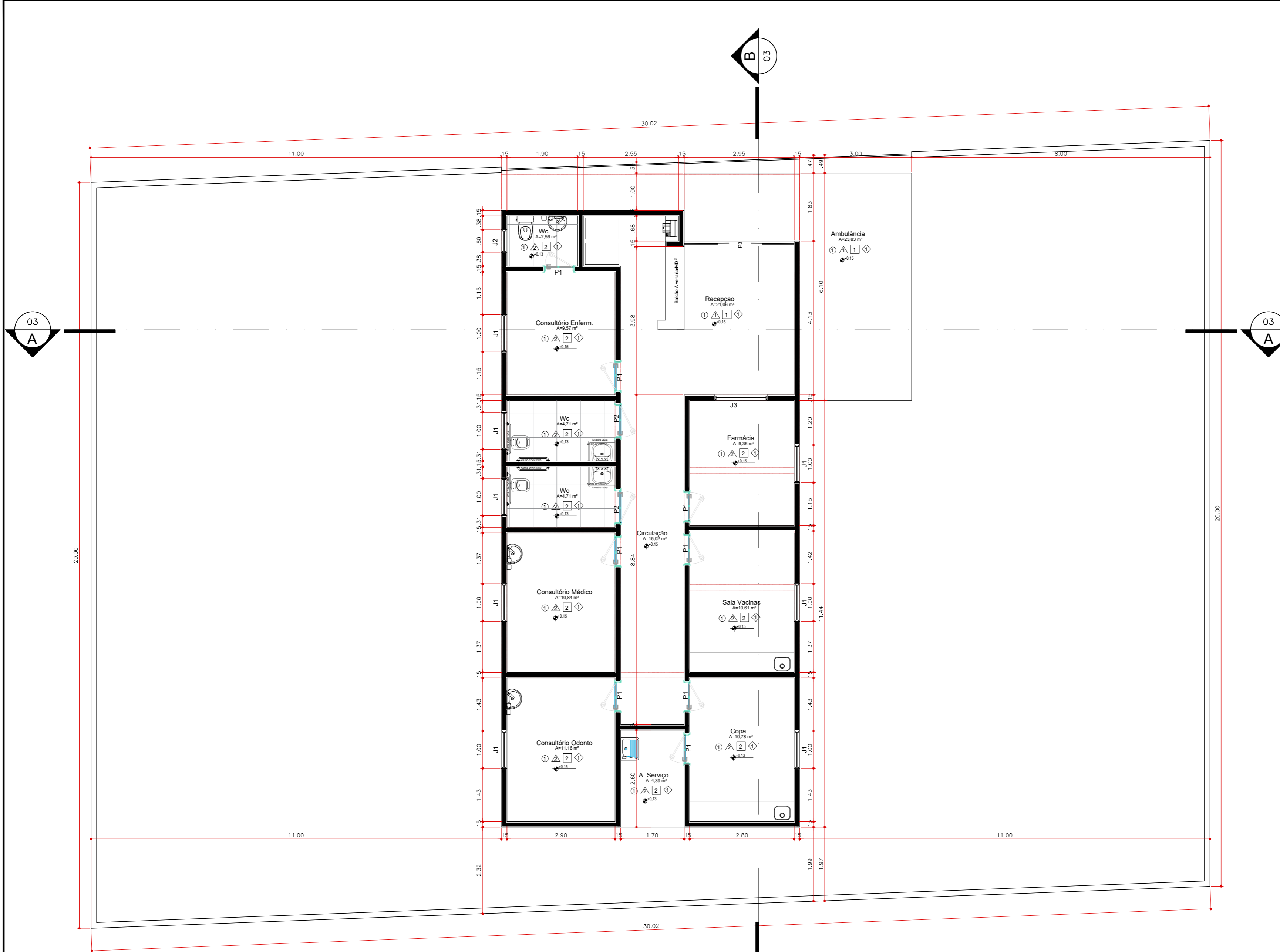
02 Planta baixa ESF Estrela do Pará 1:75
